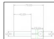
Plan d'encombrement
