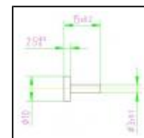
Plan d'encombrement
